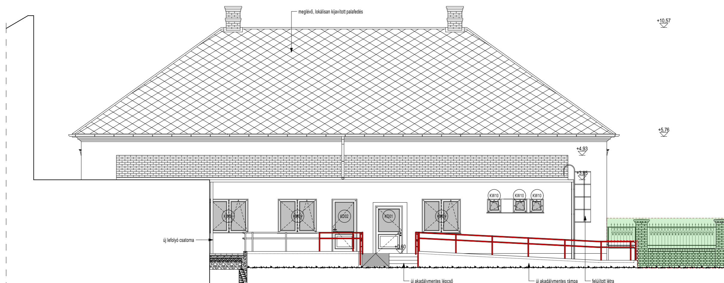
TERVEZETT NYUGATI HOMLOKZAT M= 1:100
